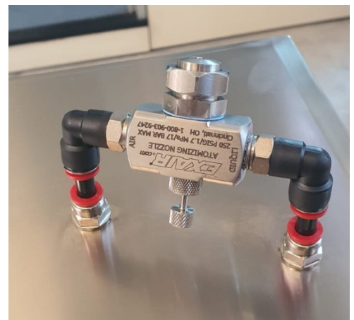
Uno degli ugelli atomizzatori EXAIR modello SR1030SS
