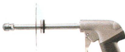
Modello 1306SS-6-CS Ugello 1006SS inox AISI 316 Prolunga alluminio 15 cm Schermo protezione in policarbonato
