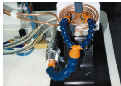
Raffreddamento trafilatura per produrre tubetti uso medicale
