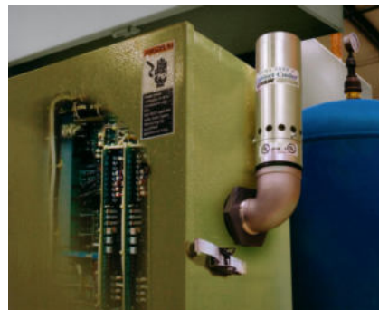
Condizionatore Exair 4630 installato sulla parete dell'armadio
