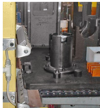
Pulizia pallet porta pezzi prima del carico del pezzo da lavorare
