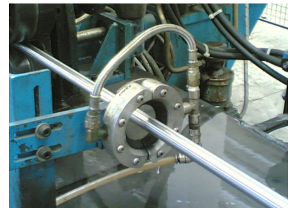
Super Air Wipe asciuga un tubo dopo la laminazione
