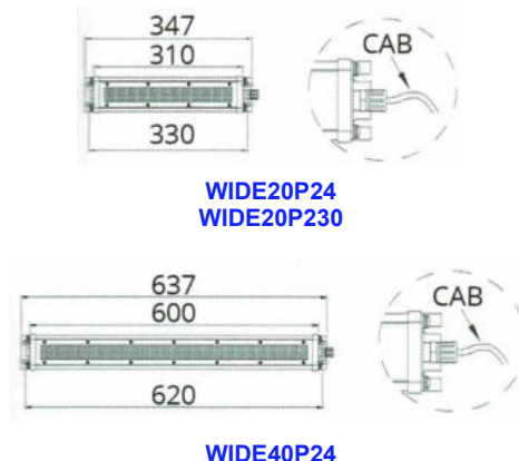
Lampade con corpo in alluminio e staffe regolabili spessore 82 mm con staffe e in posizione parallela al piano di montaggio
