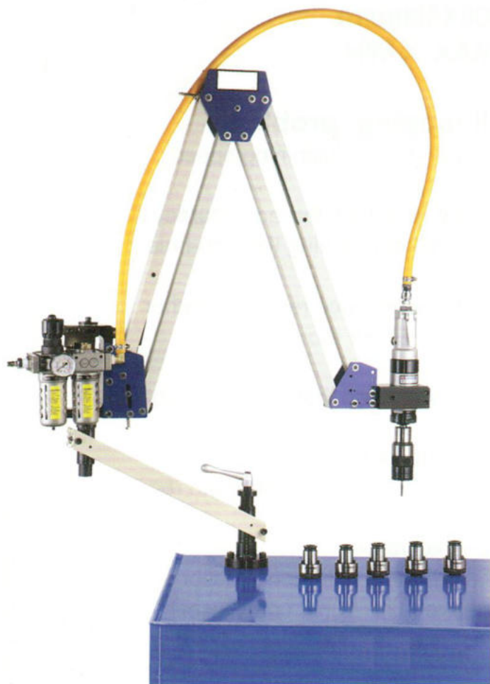
Braccio parallelo codice VAT1900 con installato maschiatore reversibile capacità da M3 a M8 codice VAT-SP08SB e gruppo filtro riduttore codice VAT-FRL con tubo aria compressa
