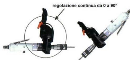
Supporto porta utensili angolare fino a 90° codice AT12-90
