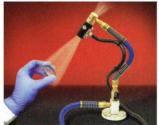
Stay Set Gen4 Ion Air Jet codice 8194-9362
