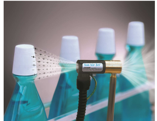
Gen4 Ion Air Jet codice 8194 neutralizza cariche su tappi di flaconi prima della stampa della scadenza e del lotto di produzione
