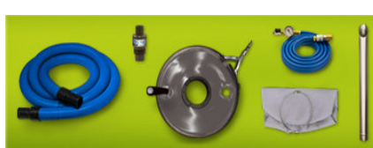
Esempio di aspiratore Heavy Duty Dry Vac per fusti da 100 e 200 litri
