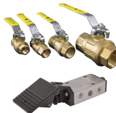
Valvole manuali a leva e a pedale per aria compressa
