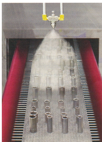
Il modello SF1020SS crea atomizzazione a cono concentrato per raffreddare o rivestire pezzi
