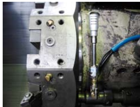
AIR LUBROCOLD installato su tornio CNC immissione direttamente nel condotto di lubrorefrigerazione della macchina (al posto dell'olio emulsionato)
