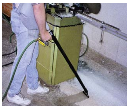
Vac-U-Gun con prolunghe in pvc e skimmer
